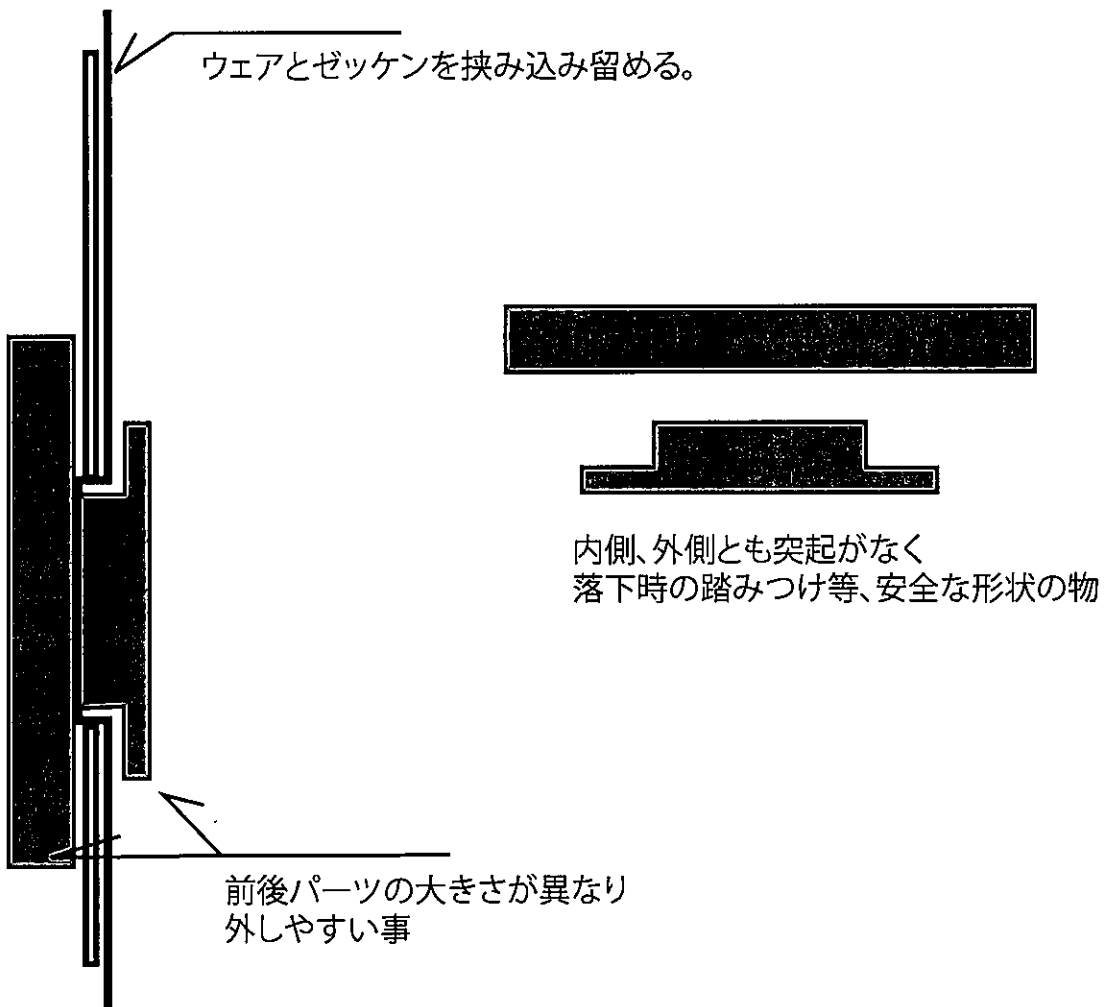
横図(拡大)
